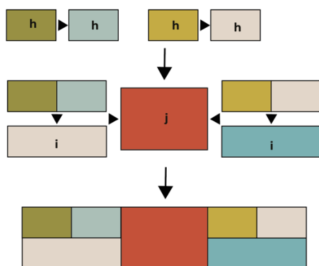
Fig. H Fabrication du Bloc 1 : partie centrale
